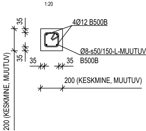
LÕIGE 1 - 1 (PIIRITÄHIS TÜÜPSARRUSTAMINE)
