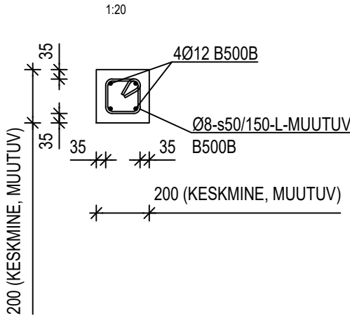
LÕIGE 4 - 4 (REKORDITÄHISE TÜÜPSARRUSTAMINE)
