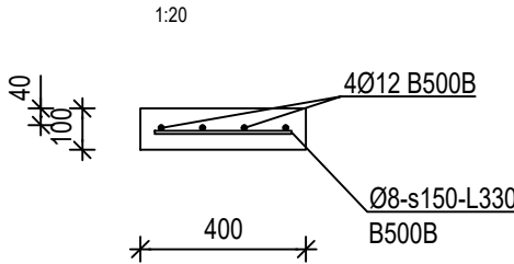
LÕIGE 2 - 2 (PIIRITÄHISE KALDKRIIPSU TÜÜPSARRUSTAMINE)
