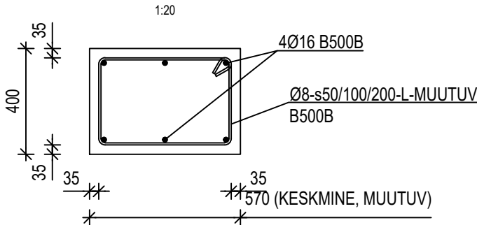
LÕIGE 3 - 3 (REKORDITÄHISE TÜÜPSARRUSTAMINE)
